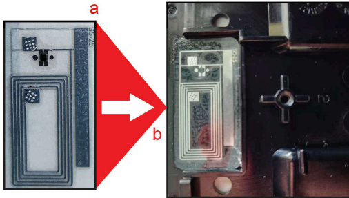
Fig. 1: RFID Tag (a), iVIZION® Cash Box (b) (P/N 272590)
